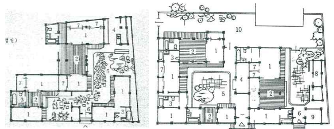
그림 1. (左) 개성 민속려관 객실 6호 평면도 (右) 객실 15호 평면도 (출처: 『조선건축』, 1990년 3호, pp.63, 57)
