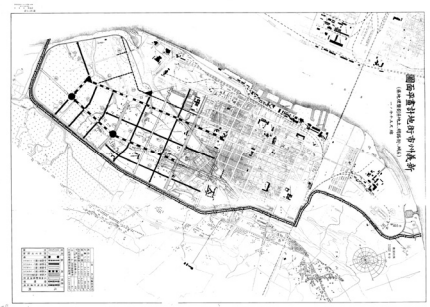
그림 4 1937년 지정된 신의주 시가지계획구역 및 간선가로망 (국가기록원 자료 CJA0003373)
