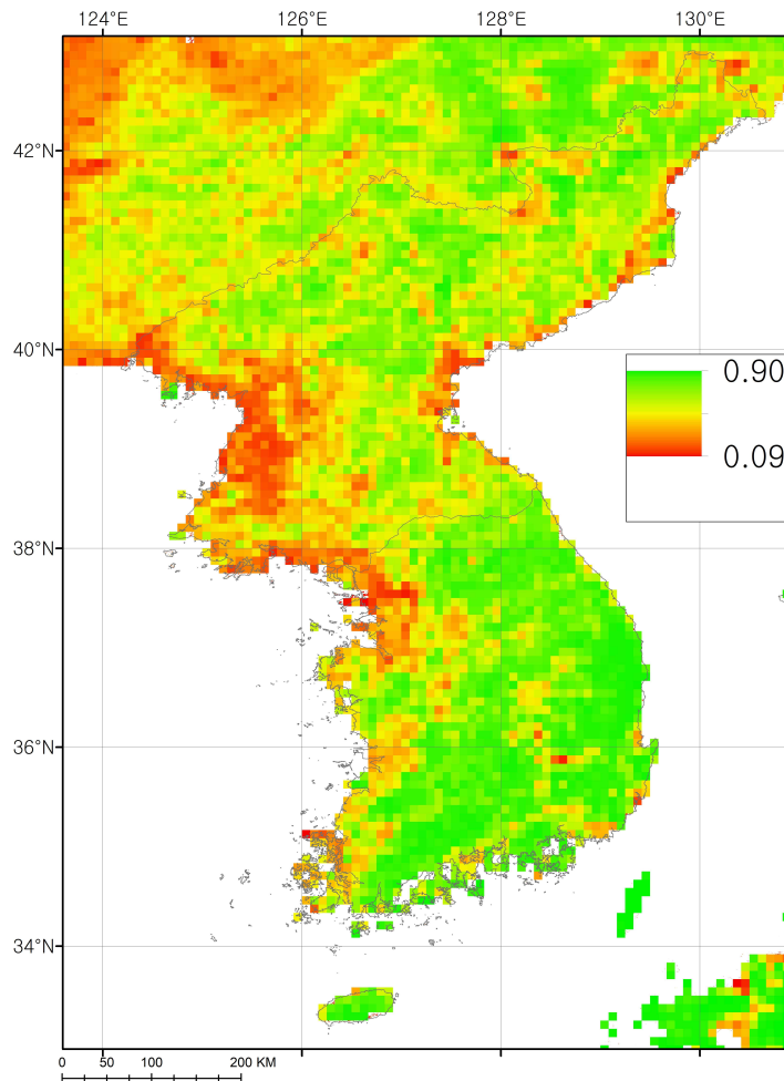
그림 7. AVHRR GIMMS NDVI 2001년 평균 예시
