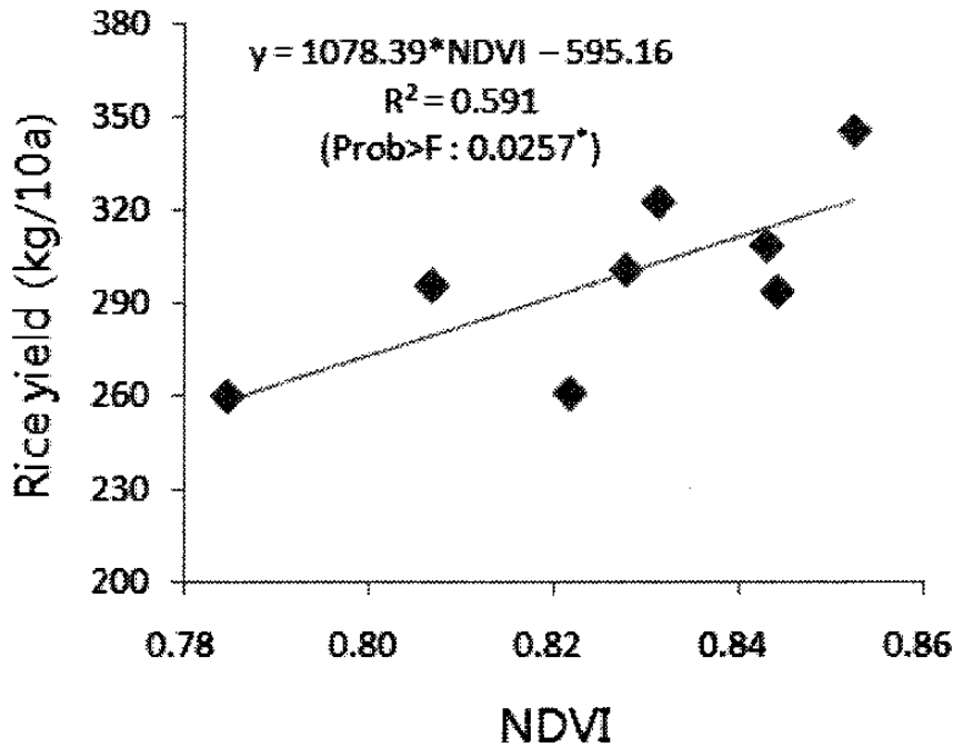
그림 2. NDVI를 이용한 식량생산량 추정모형(홍석영 등, 2009)
