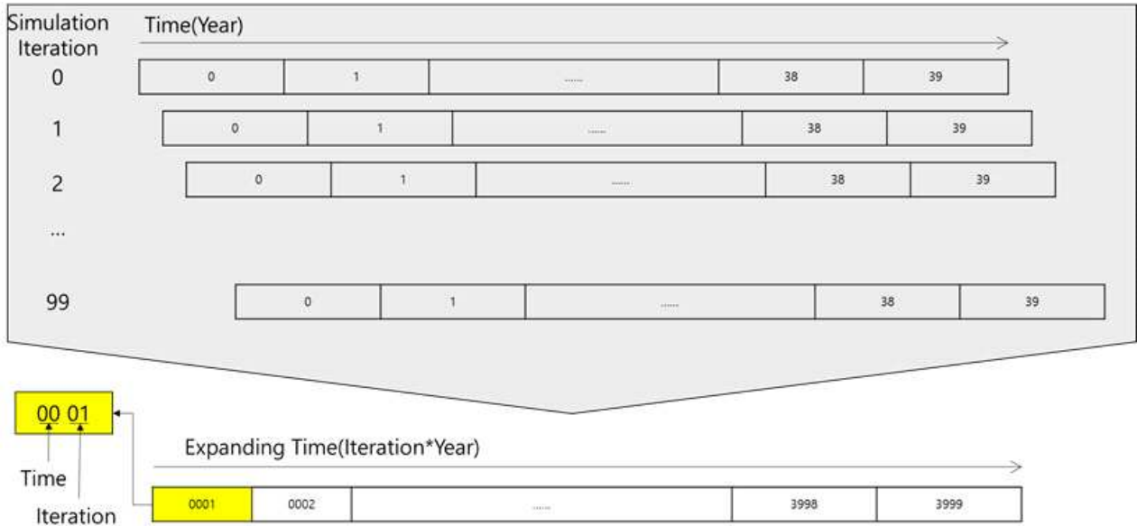
그림 28. 반복 모의결과를 시계열로 치환(“Iteration-for-Time Substitution”)하는 것의 모식도
